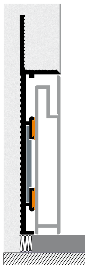
Installazione a chiusura totale Total closure installation
