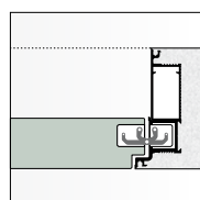
Telaio Filomuro 102 Filomuro 102 frame
