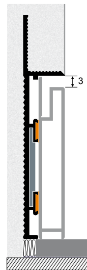
Installazione con fuga da 3 mm 3 mm leak installation
