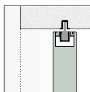
Telaio senza traverso. Frame without crosspiece.
