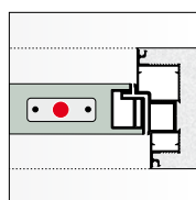
Telaio Centromuro 102 Center-Wall 102 frame
