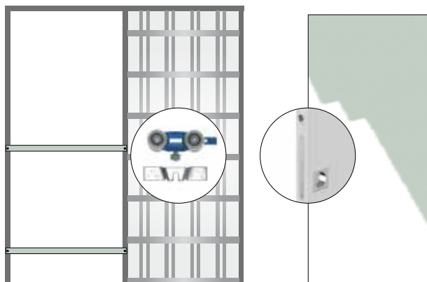
Telaio / Frame
