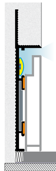
Installazione con illuminazione a led Led lightening installation
